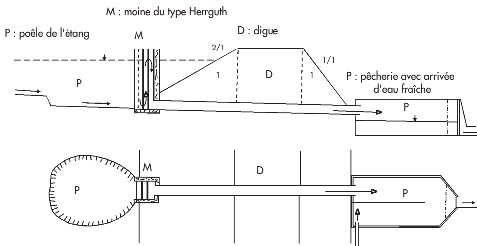
Fig. 2 – Système de vidange
